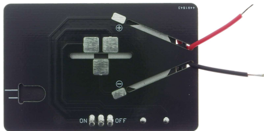
Fot. 7 Skrócone przewody koszyka baterii przed ułożeniem i przyłutowaniem do płytki podstawy
