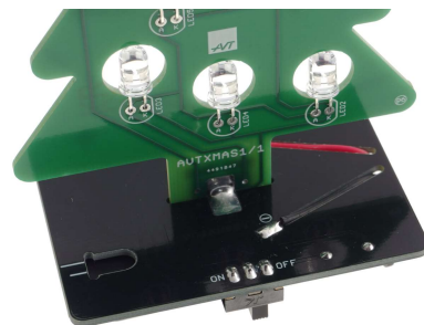
Fot. 12 Płytko choinki i podstawy po złutowaniu dodatkowego pola lutowniczego
