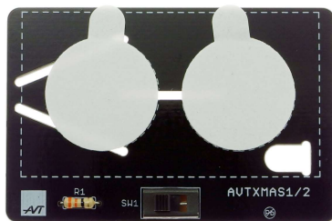
Fot. 5 Zlutowana płytka podstawy bez koszyka baterii
