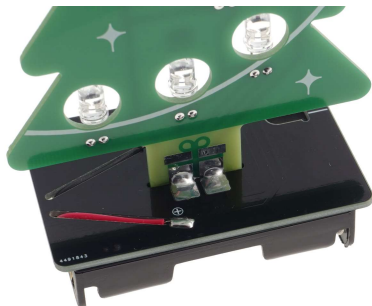
Fot. 10 Płytko choinki i podstawy po złutowaniu pól lutowniczych "prezenty"
