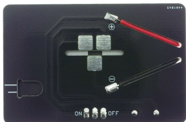
Fot. 8 Przyłutowane przewody koszyka baterii do płytki podstawy
