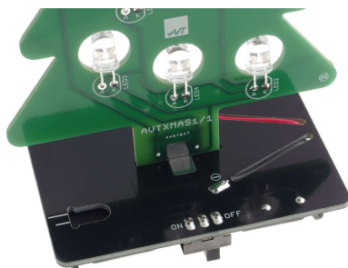
Fot. 11 Płytko choinki i podstawy przed złutowaniem dodatkowego pola lutowniczego
