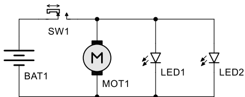
Rys. 1 Schemat ideowy
