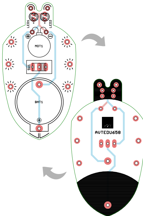
Rys. 2 Rozmieszczenie elementów na płytce drukowanej
