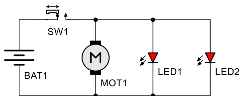
Rys. 1 Schemat ideowy
