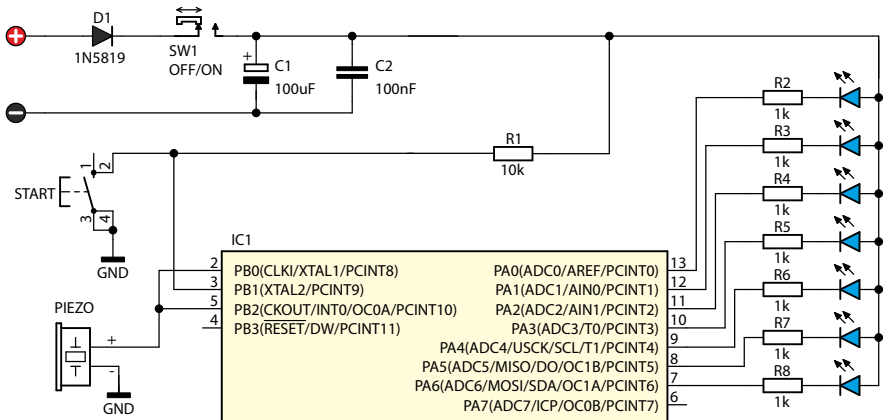
Abb. 1. Schematische Darstellung
