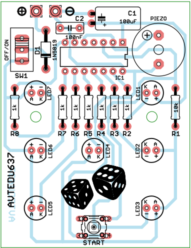
Abb. 2 Anordnung der Bauteile auf der Leiterplatte
