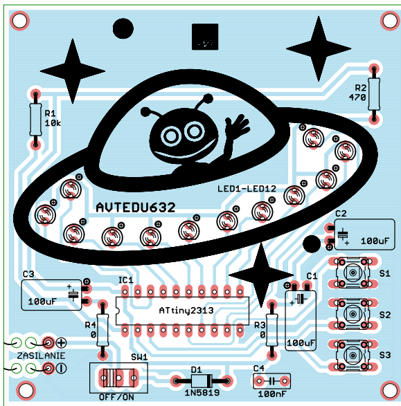
Abb. 2 Anordnung der Bauteile auf der Leiterplatte
