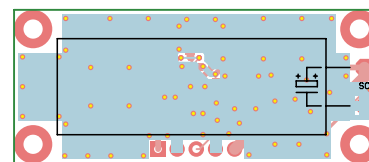
Rysunek 6. Schemat płytki PCB wraz z rozmieszczeniem elementów, strona BOTTOM
