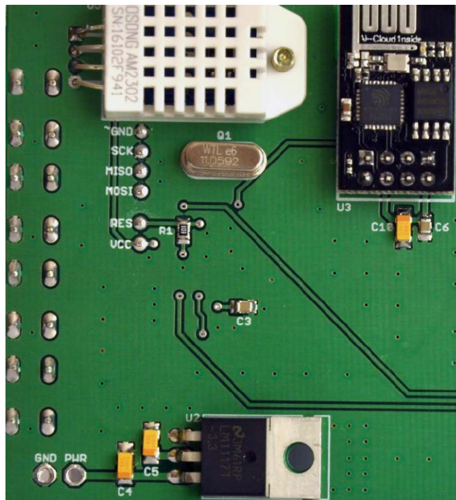
Fotografia 6. Wygląd płytki drukowanej stacji wiStation od strony wyprowadzeń
