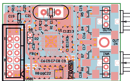
Rysunek 2. Schemat montażowy PicoDSP
