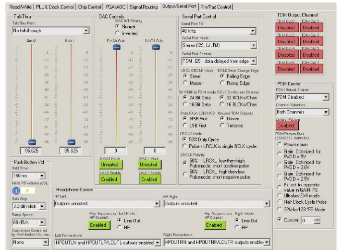
Rysunek 8. Konfiguracja przetworników C/A i sekcji wyjść
