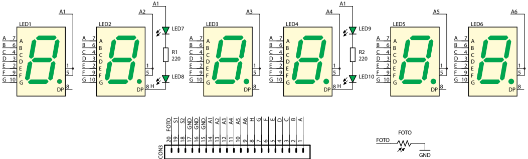
Rys. 2. Schemat ideowy wyświetlacza
