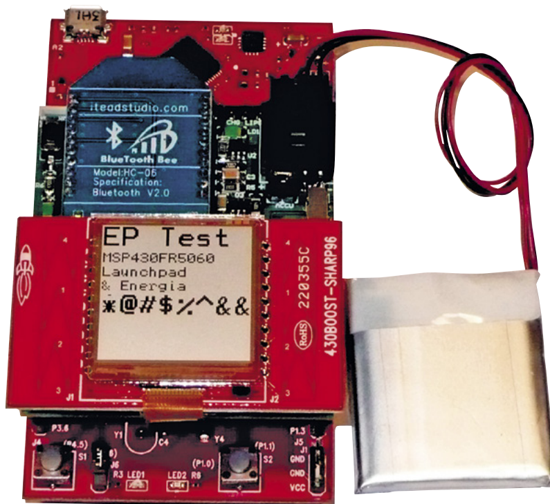
Fotografia 3. Przykładowy zestaw mobilny
