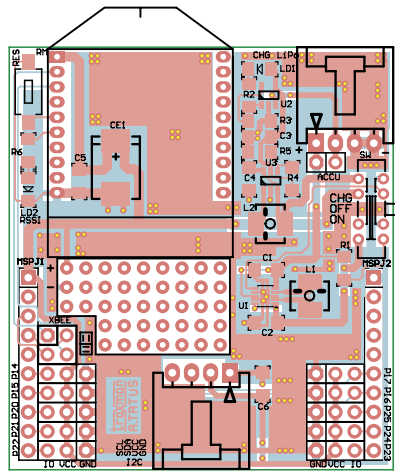
Rysunek 2. Schemat montażowy modułu zasilacza buforowego
