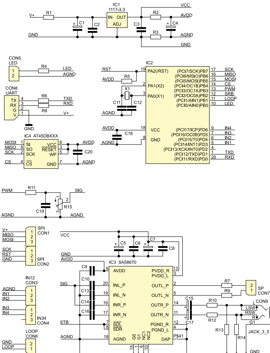
Rysunek 1. Schemat ideowy odtwarzacza
