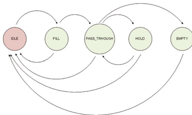
Rysunek 8. Graf pracy automatu obsługującego tryb UltraDMA
