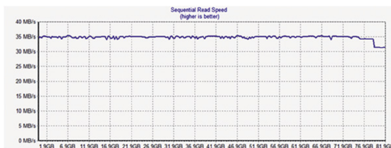
Rysunek 14. Test prędkości transferu dysku twardego Maxtor 80 GB podłączonego poprzez przejściówkę USB ↔ IDE
