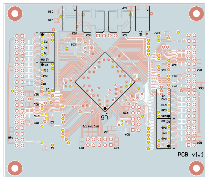
Rysunek 16. Schemat montażowy szyfrowarza
