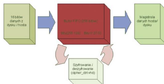
Rysunek 9. Schemat blokowy idei szyfrowania danych w FIFO
