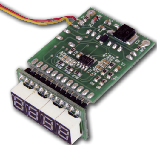
Rysunek 6. VMOD pracujący jako amperomierz
