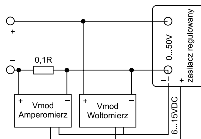
Rysunek 6. VMOD pracujący jako amperomierz
