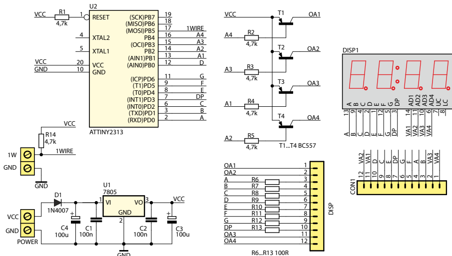
Rys. 1. Schemat ideowy
