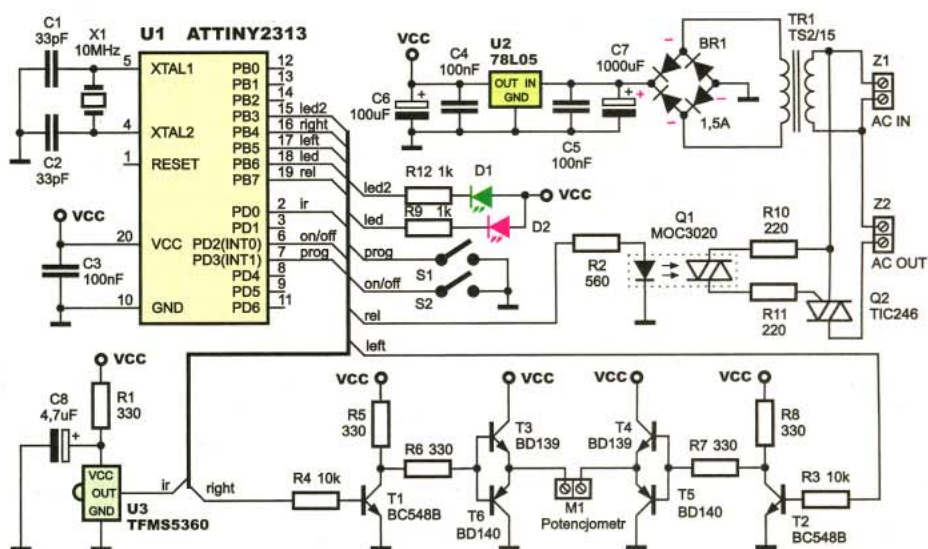
Rys. 1 Schemat ideowy
