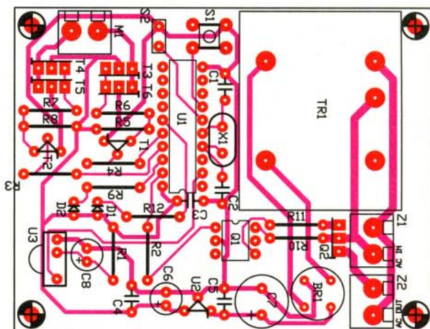
Rys. 6 Schemat montażowy
