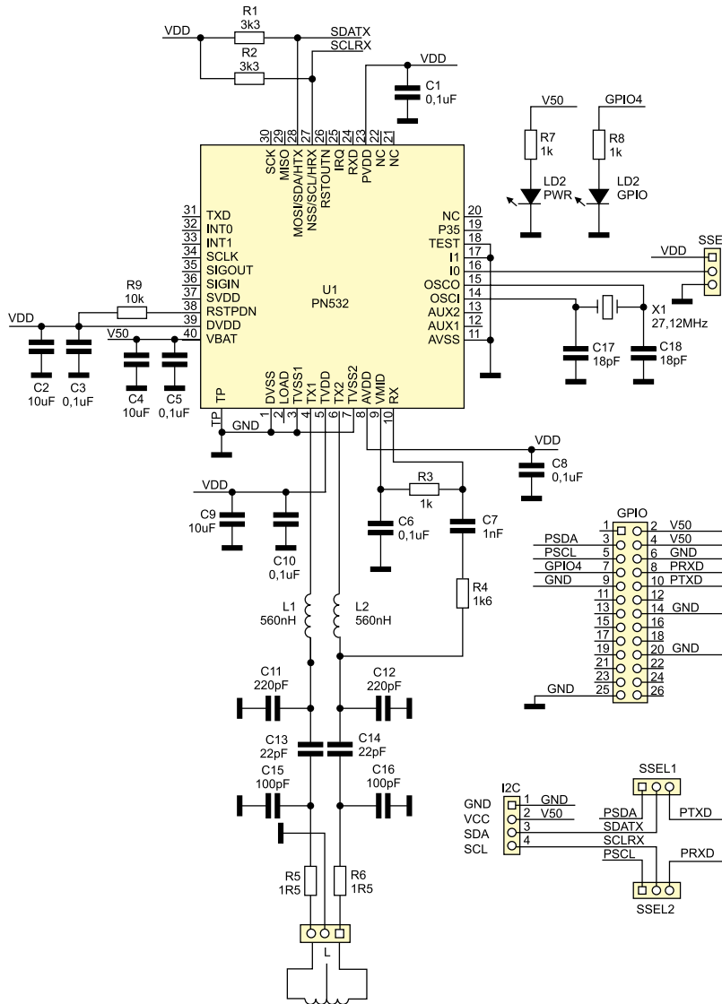
Rysunek 2. Schemat ideowy modułu RasbpI_NFC
