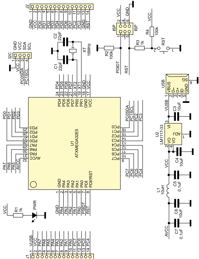
Rysunek 3. Schemat ideowy modułu x XMega32E5
