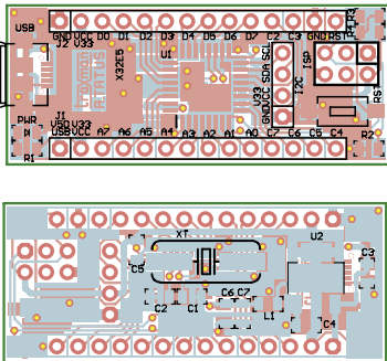
Rysunek 4. Schemat montażowy modułu x XMega32E5
