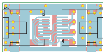
Rysunek 2. Schemat montażowy zabezpieczenia RJ45
