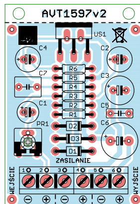
Rys. 2. Rysunek montażowy
