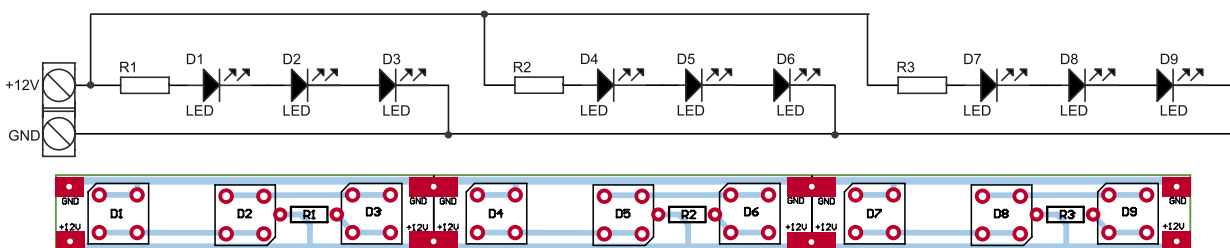
Rys. 1c. AVT1502 – 1x9LED
