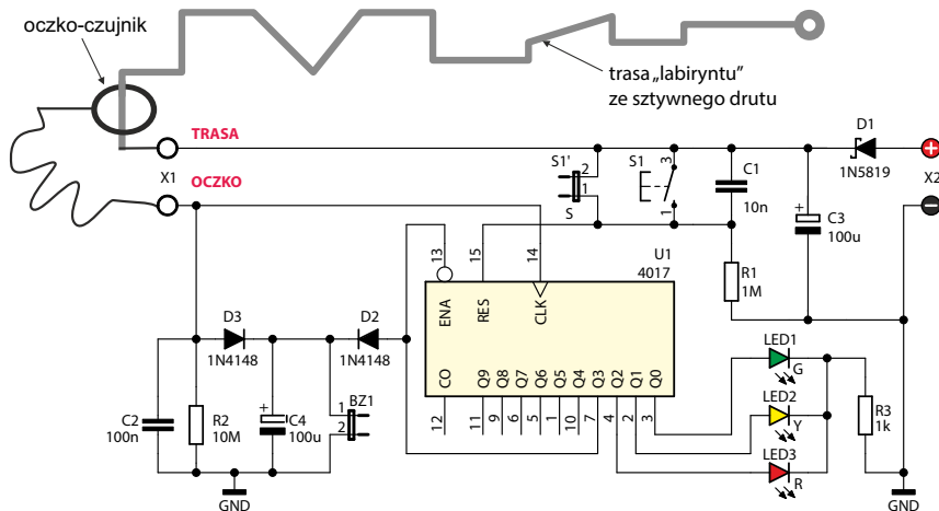
Rys. 1 Schemat ideowy
