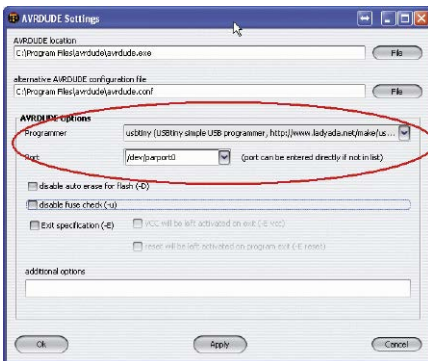
Rysunek 4. Wybór rodzaju programatora
