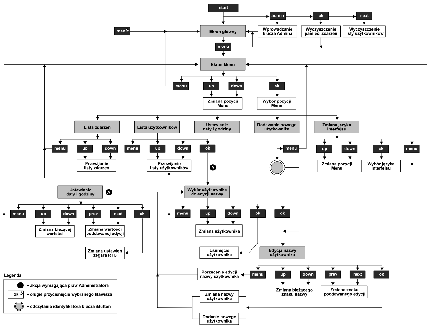
Rysunek 3. Diagram prezentujący kompletny algorytm obsługi systemu menu sterownika systemu SAS
