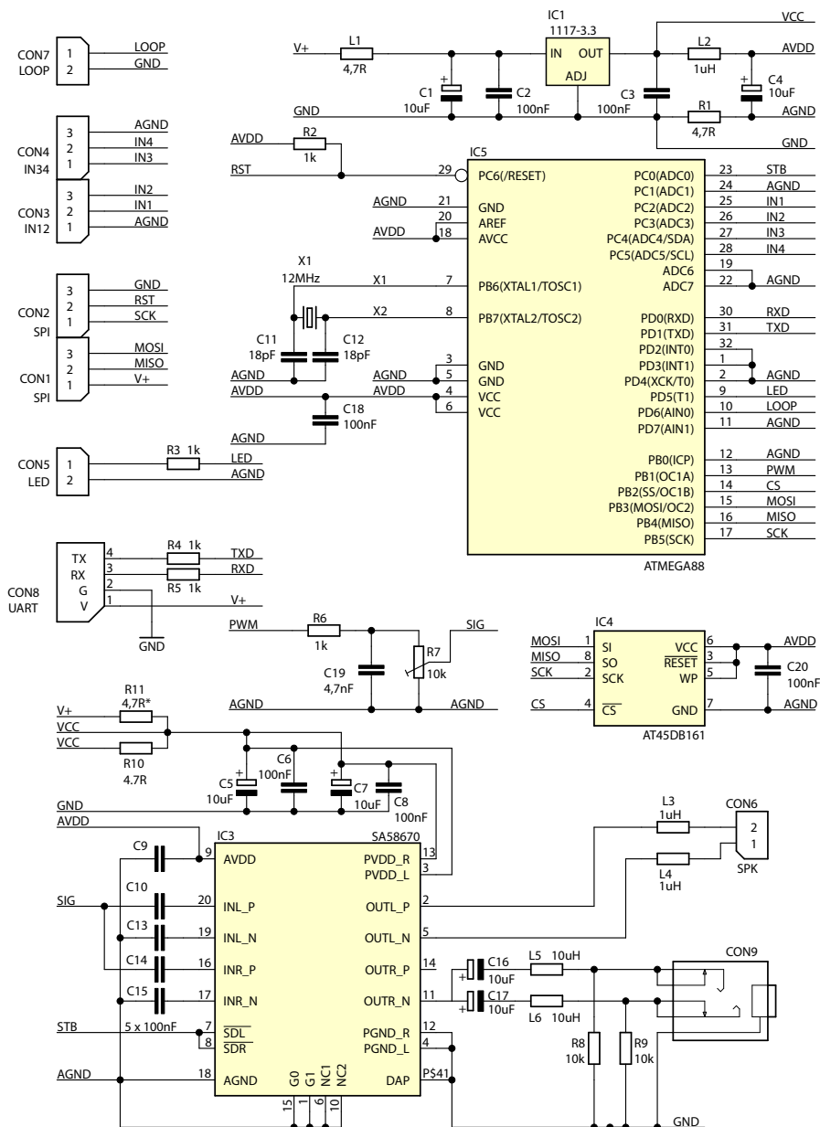
Rysunek 1. Schemat ideowy odtwarzacza
