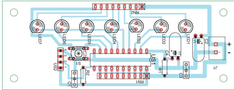
Rysunek 2. Schemat montażowy higrometru
