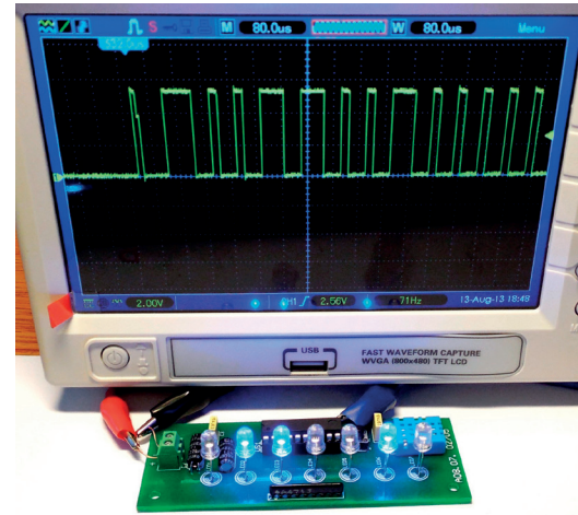
Fotografia 5. Zestawienie wskaźników układu z oscylogramem
