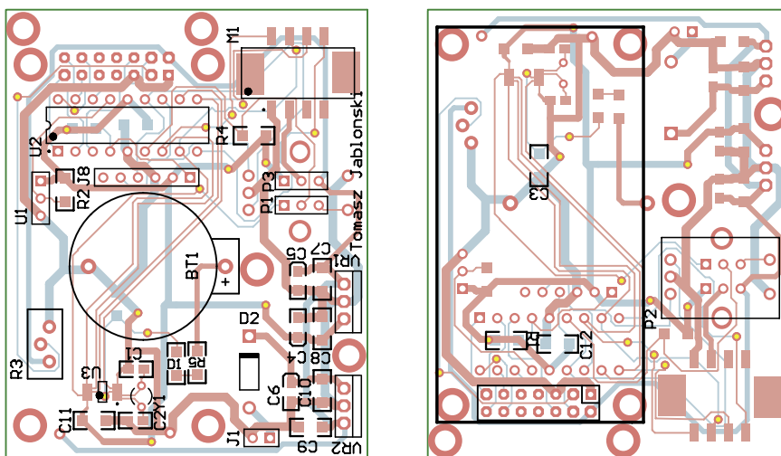
Rysunek 2. Płytkę drukowaną zegara z termometrem
