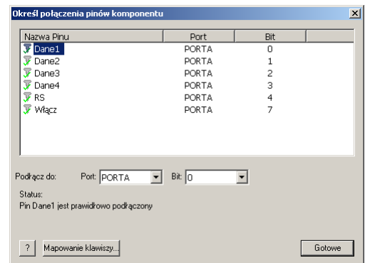
Rysunek 4. Okno definicji połączeń wyświetlacza LCD
