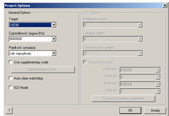
Rysunek 6. Ustawienie częstotliwości taktowania dla symulatora oraz procedur odmierzenia czasu
