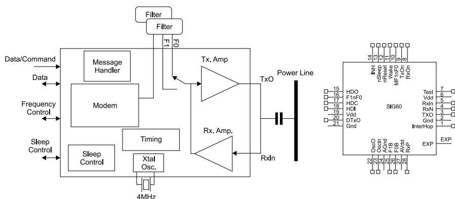
Rysunek 3. Struktura wewnętrzna układu SIG60 oraz jego wyprowadzenia
