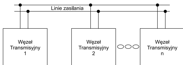
Rysunek 2. Struktura sieci PLC w topologii magistrali
