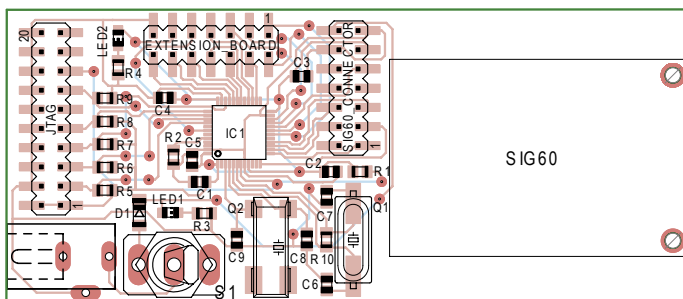
Rysunek 7. Rozmieszczenie elementów na płytce drukowanej węzła komunikacyjnego
