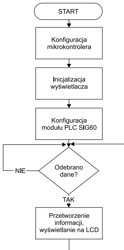
Rysunek 6. Schemat blokowy programu węzła odbiorczego
