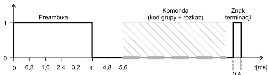
Rys. 9. Ramka danych przyjęta w standardzie Technics
