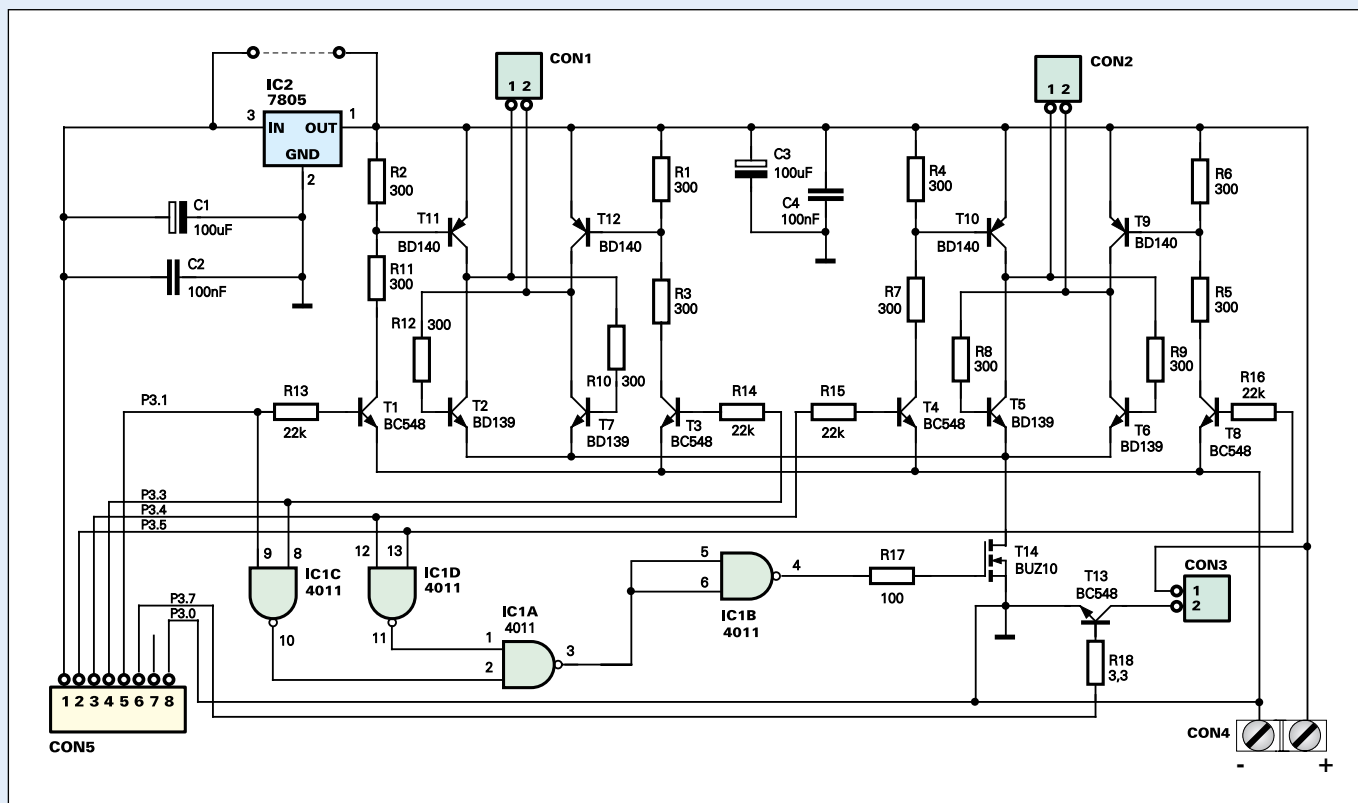
Rys. 2 Część wykonawcza
