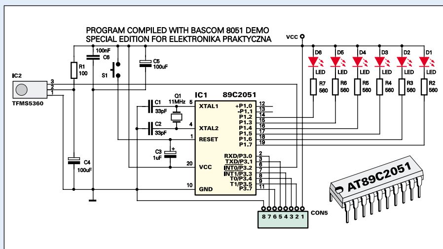
Rys. 1 Sterownik
