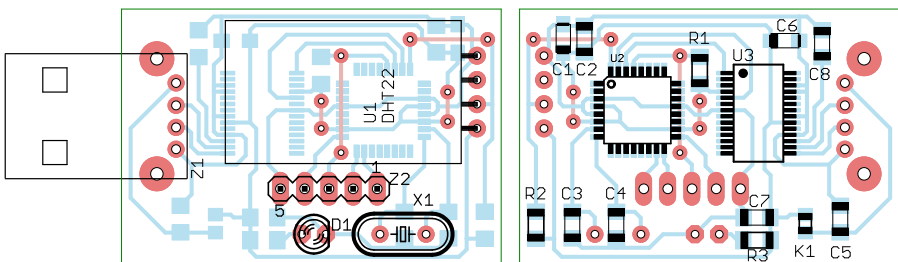
Rysunek 4. Schemat montażowy termometru
